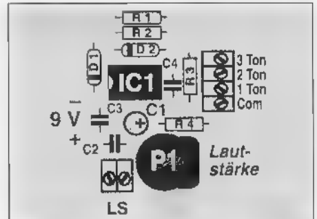
Figuur 2: De componentenopstelling van de HB409.
